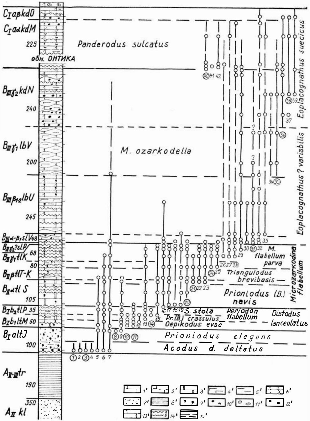
Рис. 1. Стратигический разрез онтикаской подсерии и азербайджанского горизонта. Условные обозначения. Известняки: 1' — горизонтально-слоистые, 2' — комковатые; 3' — доломиты, 4' — мергели, 5' — глинистые породы, 6' — песчаники, 7' — пески оболовые, 8' — аргиллиты коричневые, 9' — глауконит, 10' — оолиты железистые, 11' — оолиты фосфатные, 12' — пирит, 13' — известняки детритовые, 14' — поверхности перерыва, (a — ровные, б — неровные), 15' — границы стратиграфических подразделений. Распределение конодонтов (номера в кружках указывают на руководящие формы): 1 — Paltodus deltifer , 2 — Drepanoistodus acuminatus , 3 — Acodus deltatus
