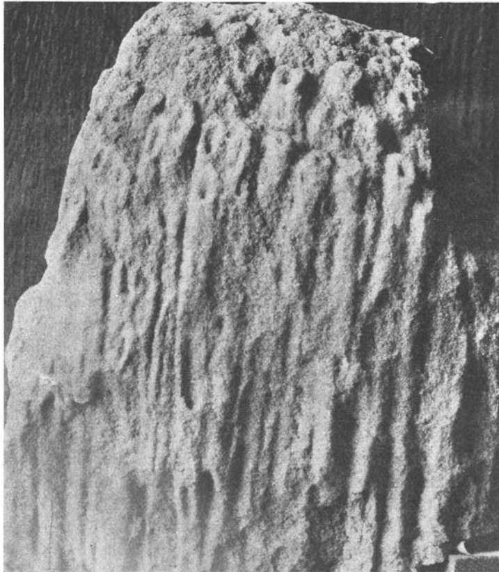
Fig. 1. Scolithussandstein. Geschiebe, Büchen.
